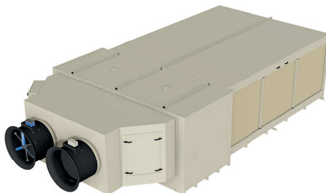
Munters LAVAMATIC® с биофильтром
