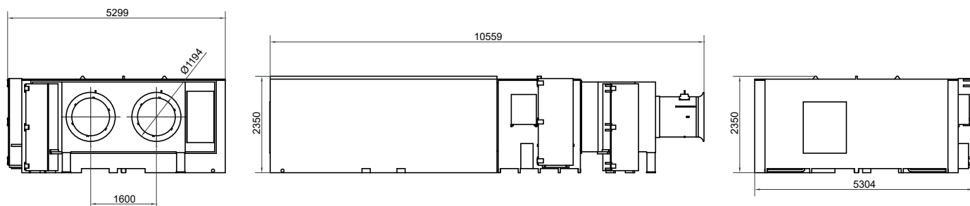
Очиститель Munters LAVAMATIC® с биофильтром
