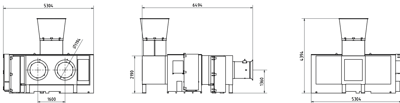
Munters LAVAMATIC® – система с модулем вытяжного воздуха
