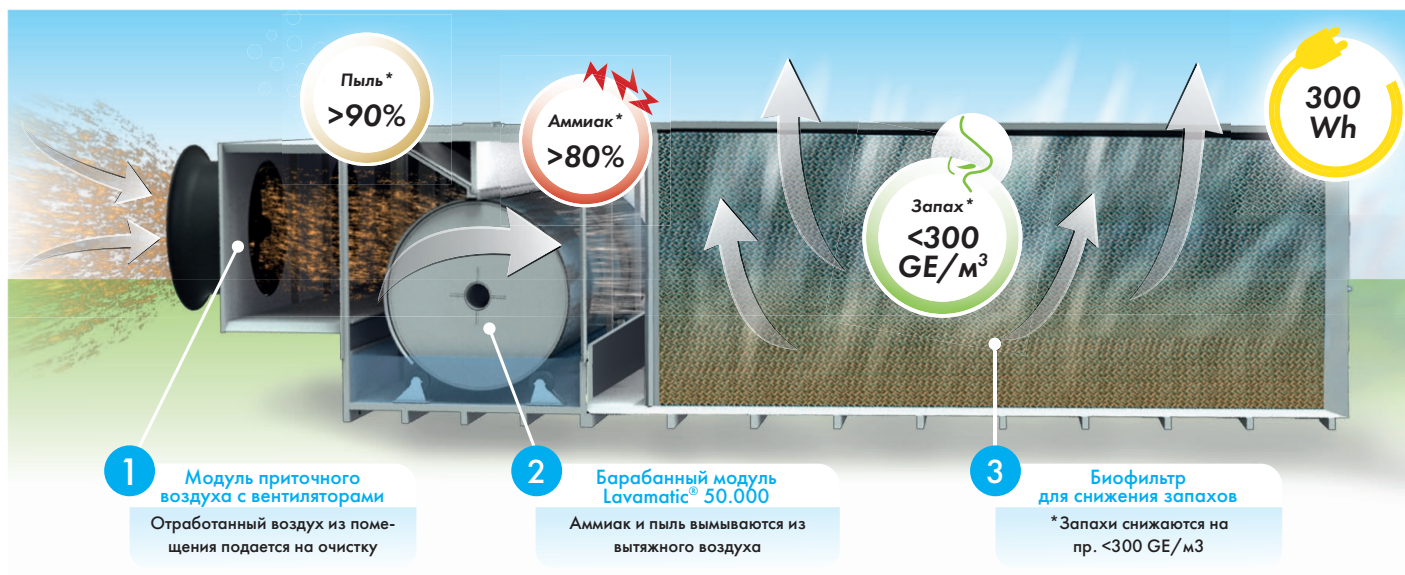
Munters LAVAMATIC® с биофильтром
