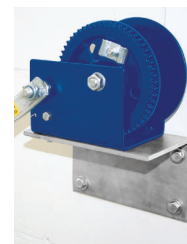
Konsolen für Seilwinde
